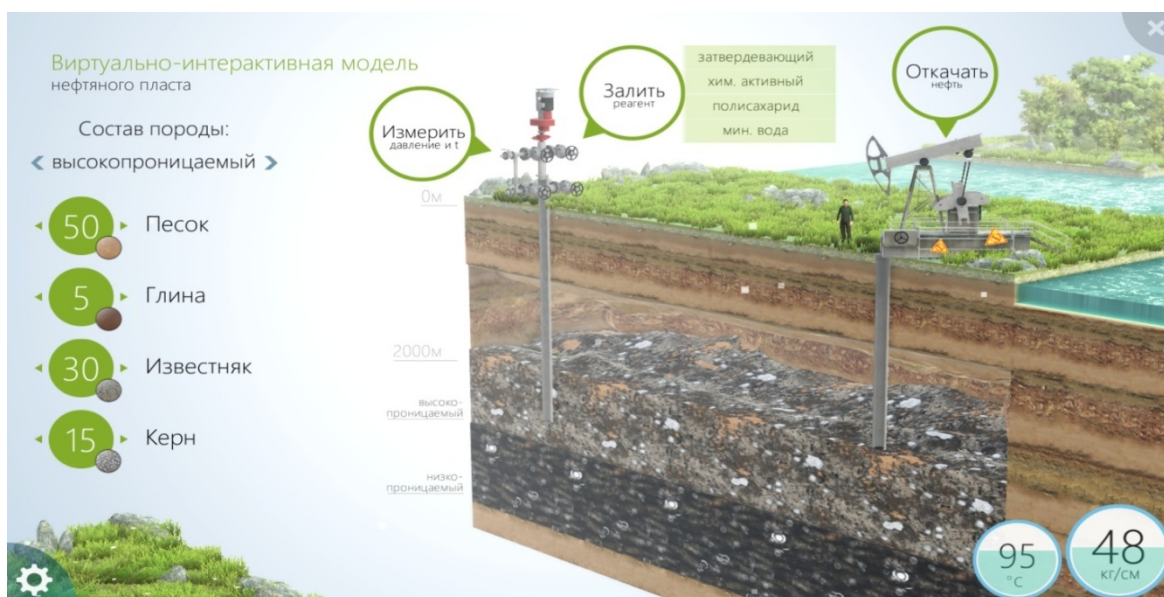
Рисунок 2–Тампонирующее высокопроницаемого канала полимером «полисах» и заводнение низкопроницаемого канала фильтрации
