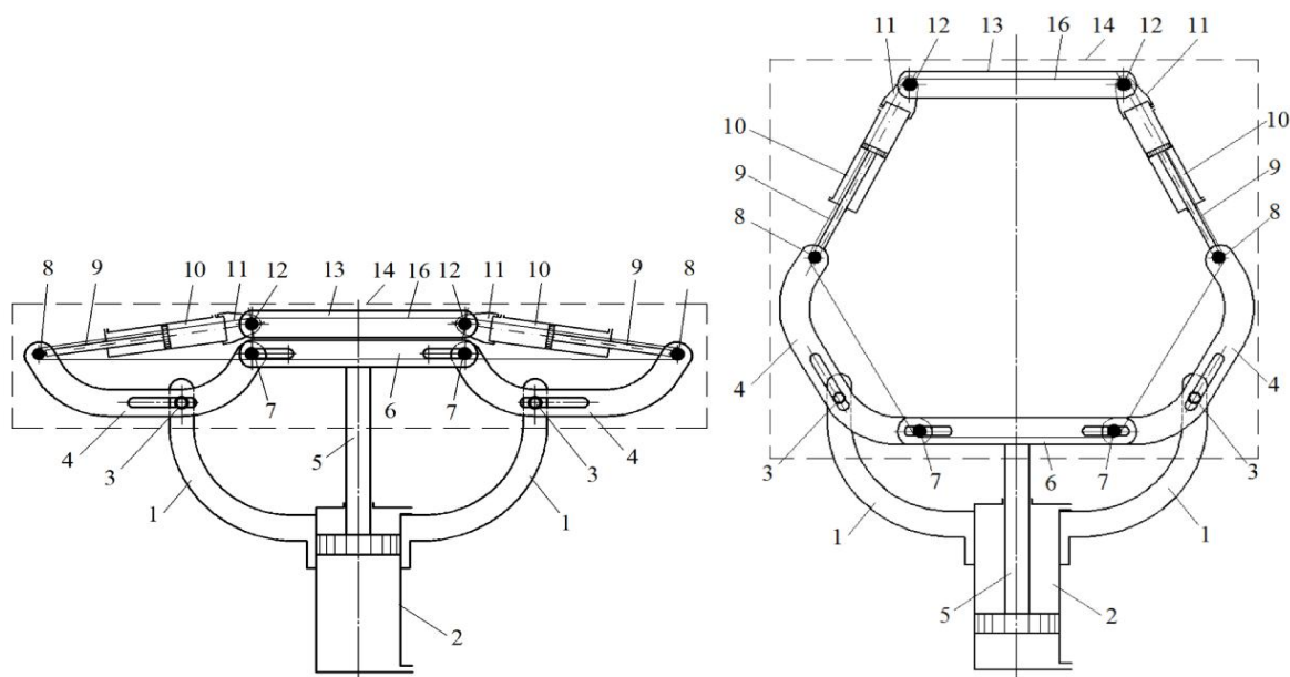
Рисунок 2 – Рычажно-шарнирное захватное устройство в двух положениях: a – в закрытом, мешок удерживается пальцами; б – в раскрытом, мешок открыт
