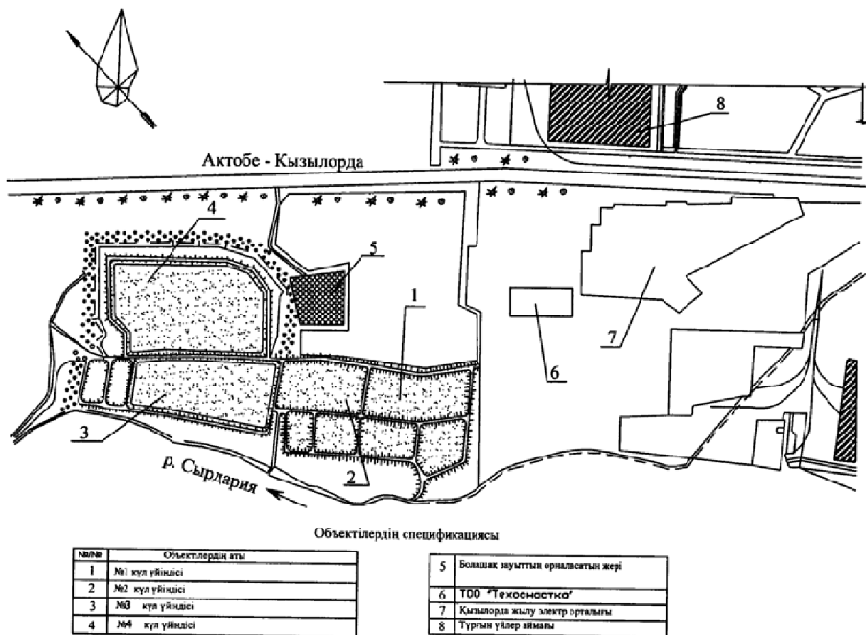
2-сурет – Қызылорда ескі күл үйінділерінің ситациялық схемасы
