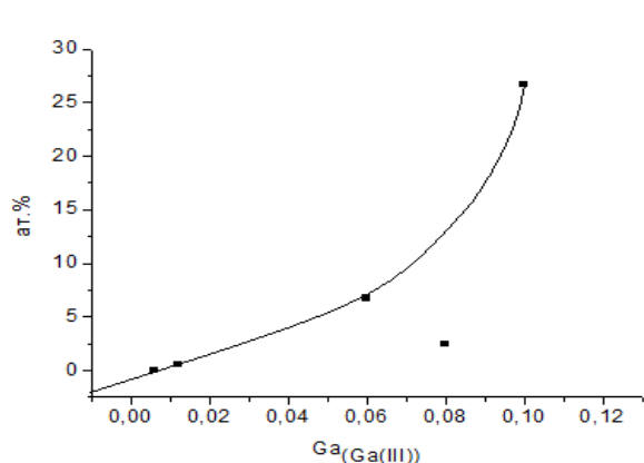
Рисунок 6 – Зависимость содержания галлия в осажденной пленке от концентрации ионов галлия в электролите при постоянном потенциале -0,8 и концентрации \text{Se} = 2 \cdot 10^{-3} \text{ M}
