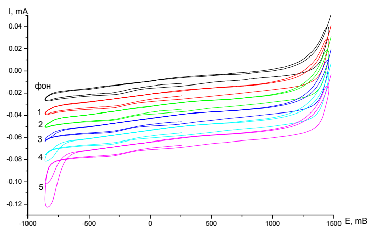
Рисунок 2 – ЦВА стеклоглеродного электрода в сернокислом электролите при различном содержании ионов галлия Ga(III) 1\cdot 5\cdot 10^{-4} ; 2\cdot 1\cdot 10^{-3} ; 3\cdot 2\cdot 10^{-3} ; 4\cdot 5\cdot 10^{-3} ; 5\cdot 1\cdot 10^{-2} М
