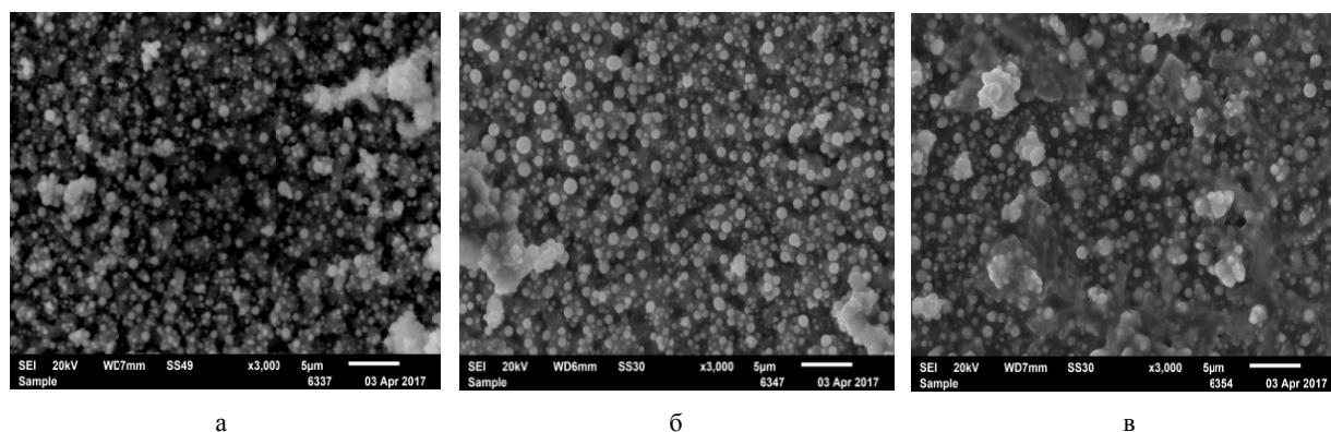
Рисунок 5 – Микрофотографии поверхности пленок: а) E_{oc} = -0,9\text{В} на СУ – 110; б) E_{oc} = -0,9\text{В} на СУ – 111; в) E_{oc} = -0,8\text{В} на СУ – 112
