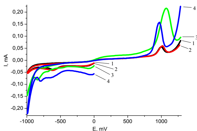
Рисунок 3 – ЦВА стеклоглеродного электрода в цитратном буферном растворе при постоянной концентрации ионов селена и различных концентрациях галлия. 1-4) Se(IV)= 2\cdot 10^{-3} М; Ga(III): 1) 6\cdot 10^{-3} ; 4) 1,2\cdot 10^{-2} ; 5) 6\cdot 10^{-2} ; 6) 8\cdot 10^{-2} М
